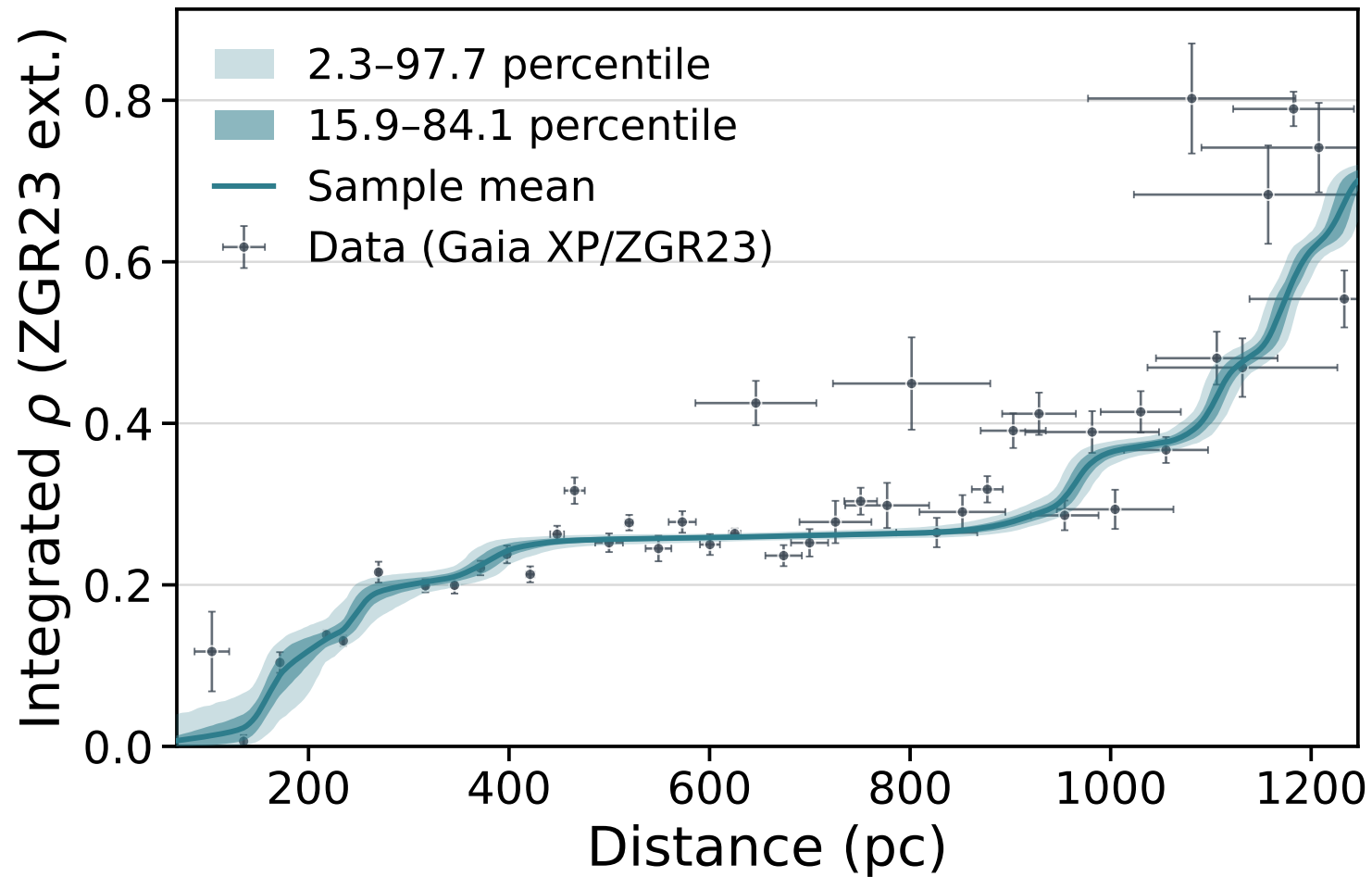
HMC posterior samples
